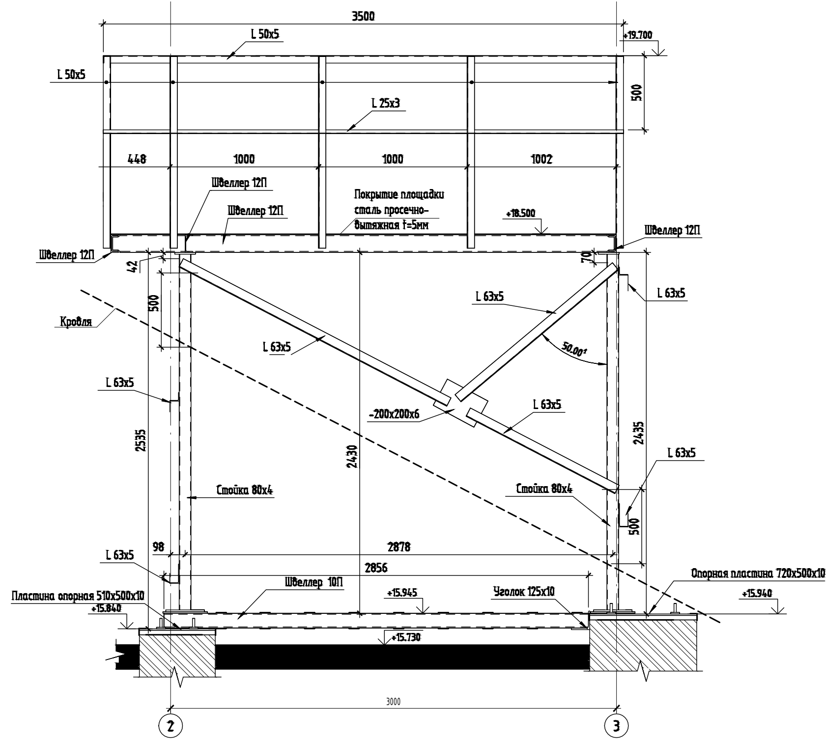
Вид 1 (1:20)
