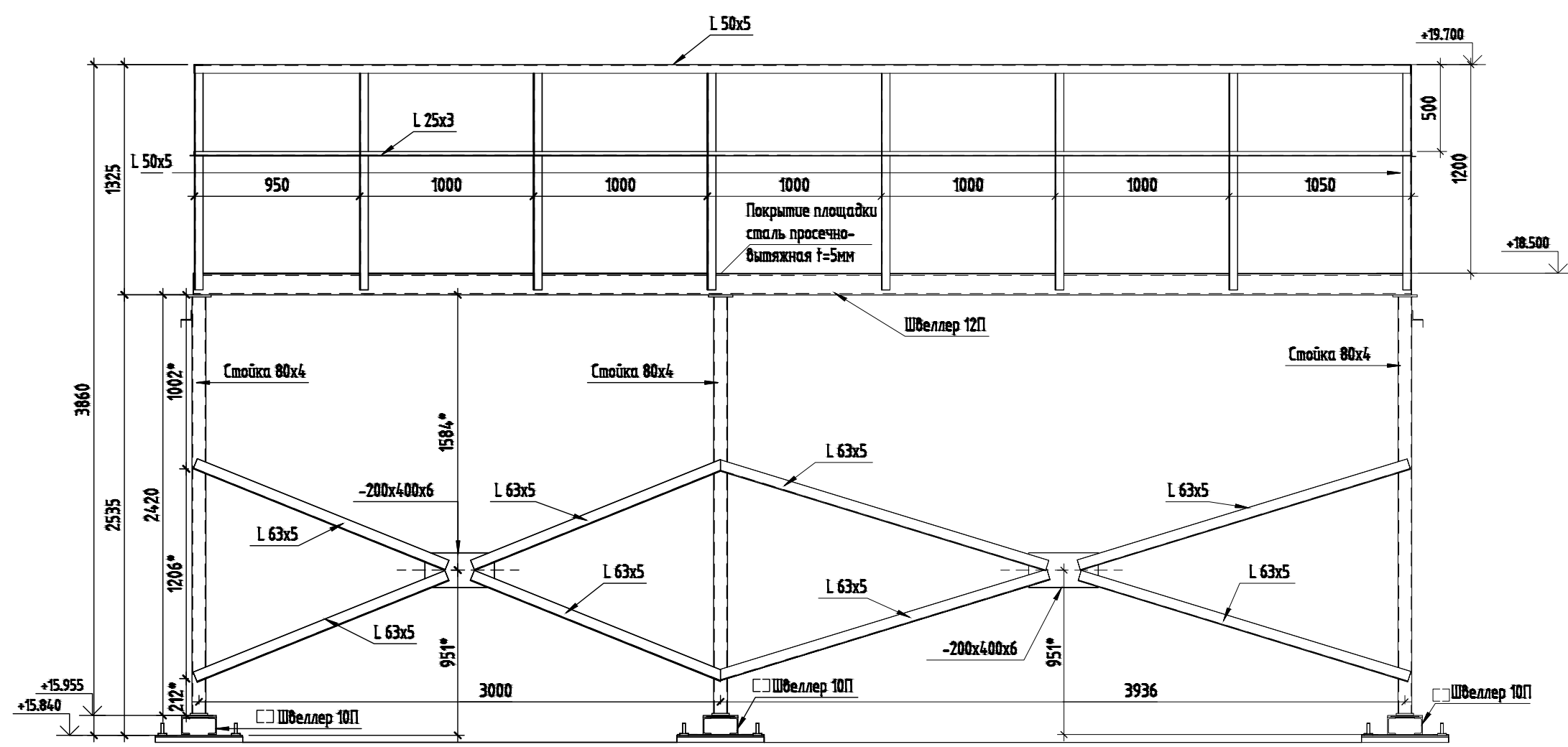
Вид 3 (1: 20)
