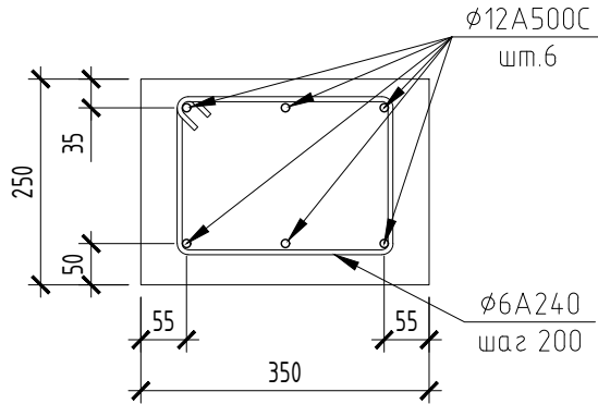
Опорная плита Оп1 Армирование
