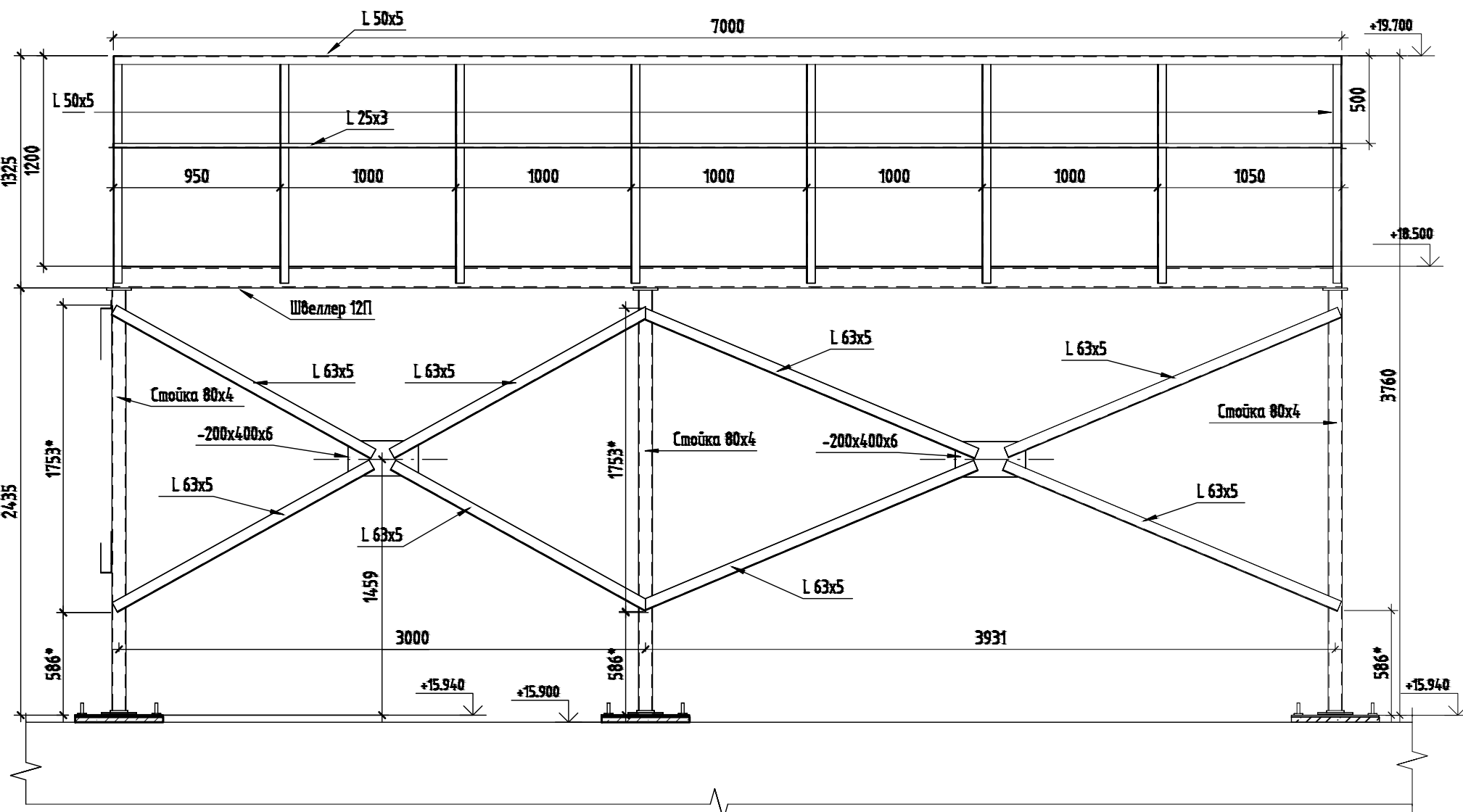
Вид 4 (1:20)
