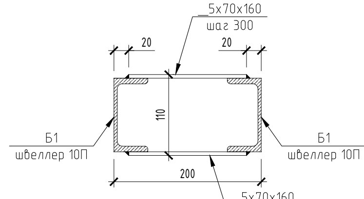
1-1 (М1:5)
