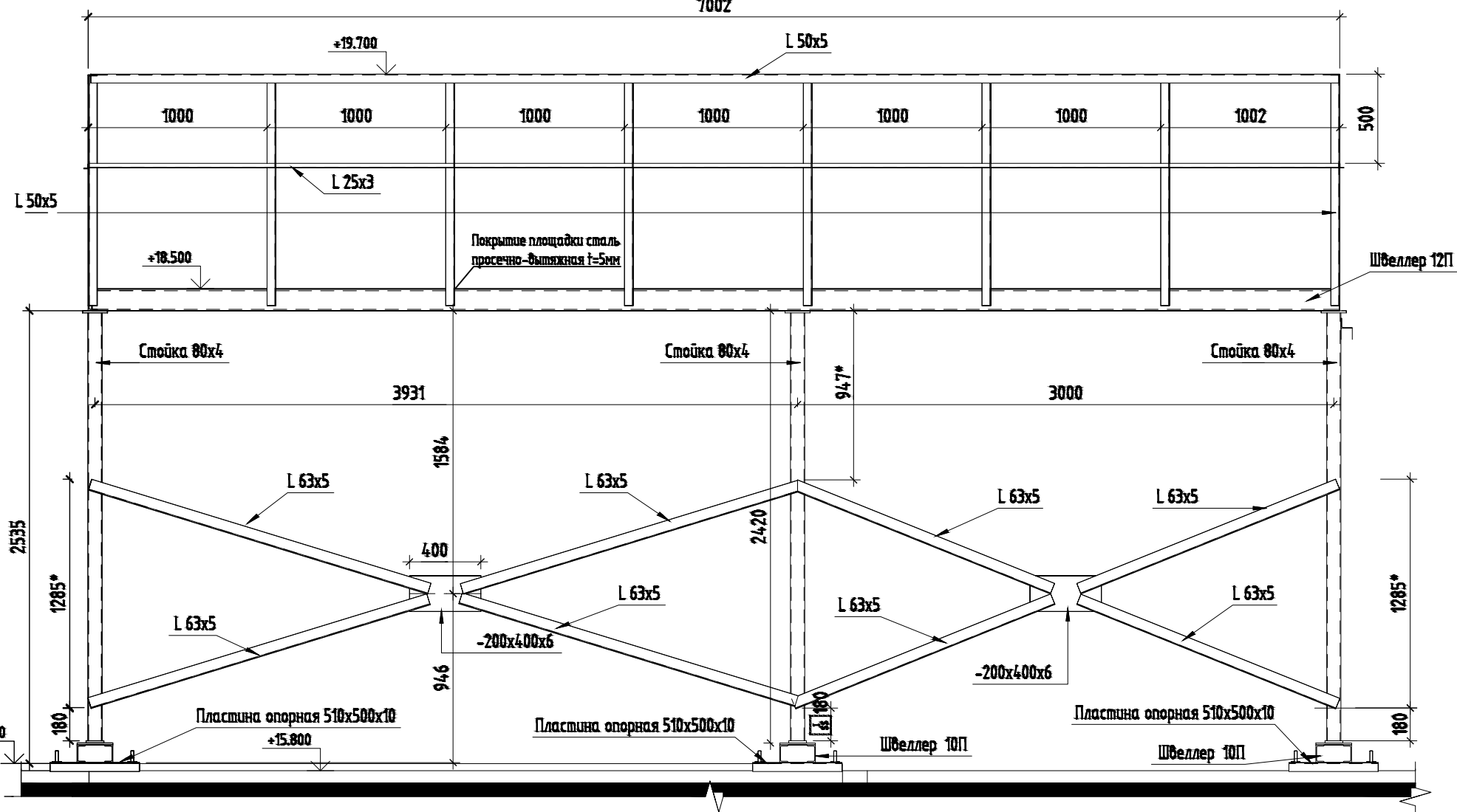
Вид 3 (1:20)
