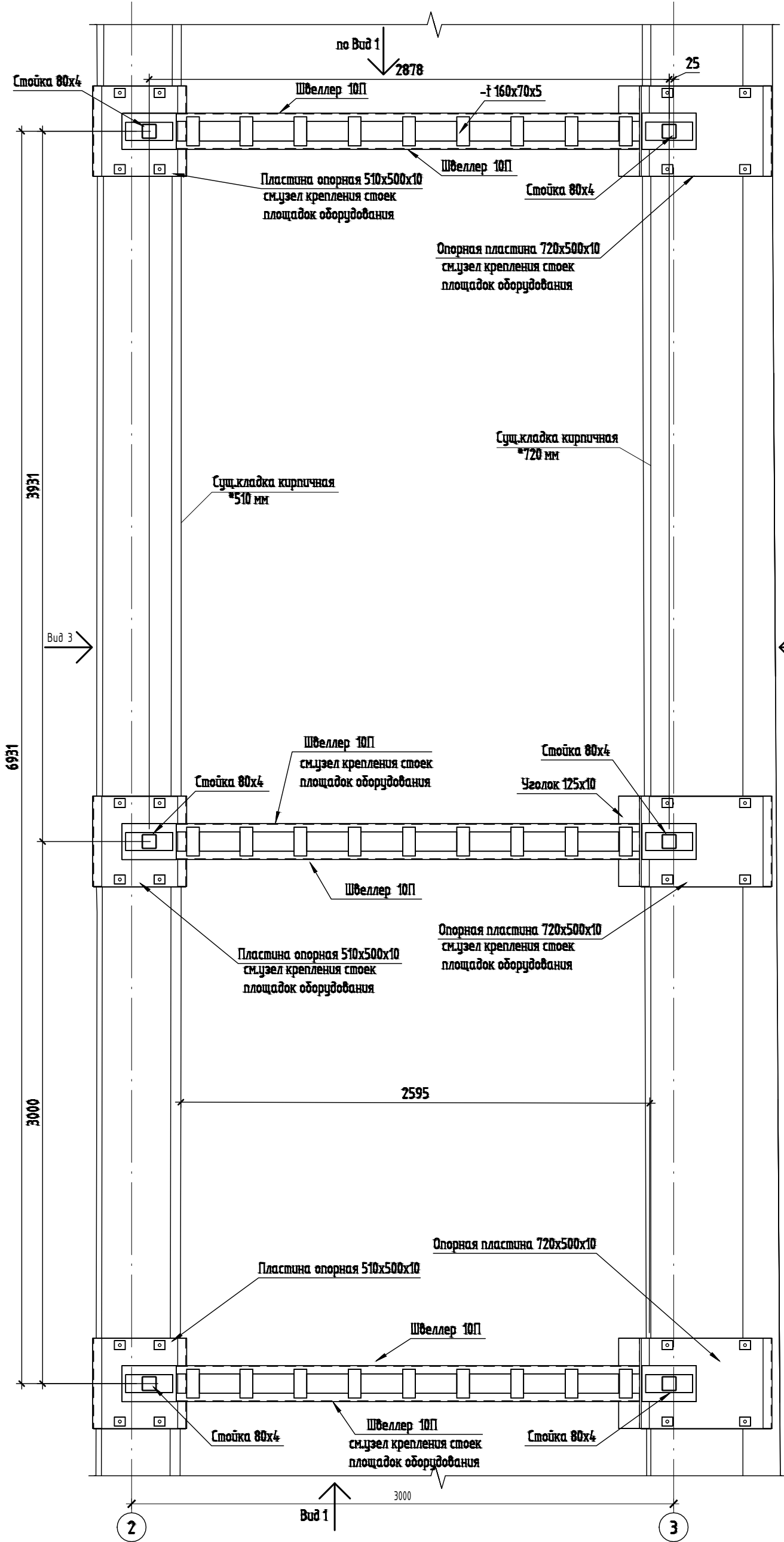
План опорных пластин и стоек под площадку Пл-1 (1:20)
